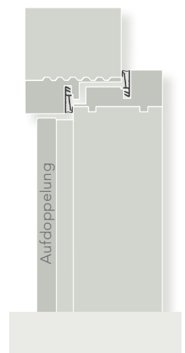
Schallschutzaufdoppelung bei Rubner KlimaHausTüren
